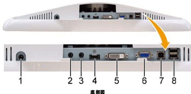
底部図
